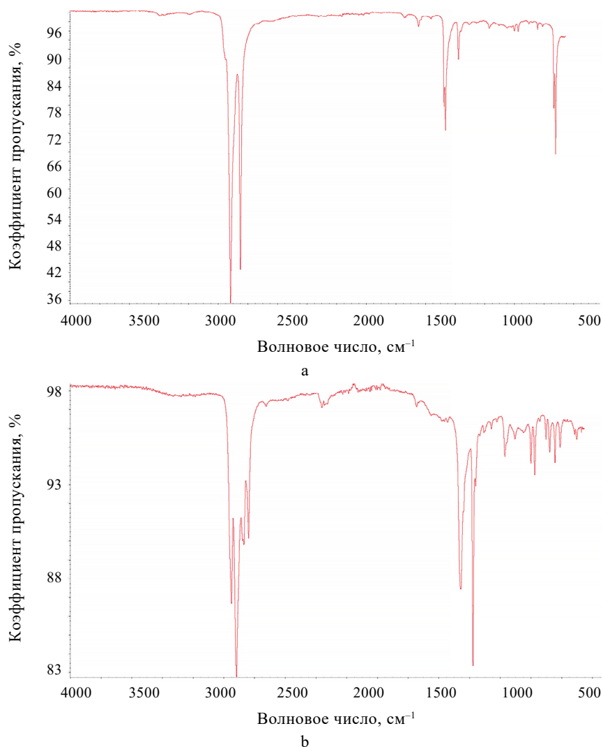
Рисунок 4. ИК-спектры исходных полиэтилена низкой плотности (а) и изотактического полипропилена (b)
