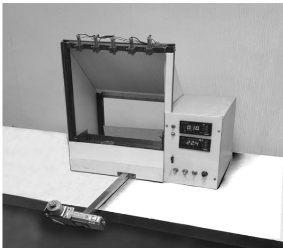
Рис. 3. Общий вид установки для исследования процесса свертывания молочных смесей
