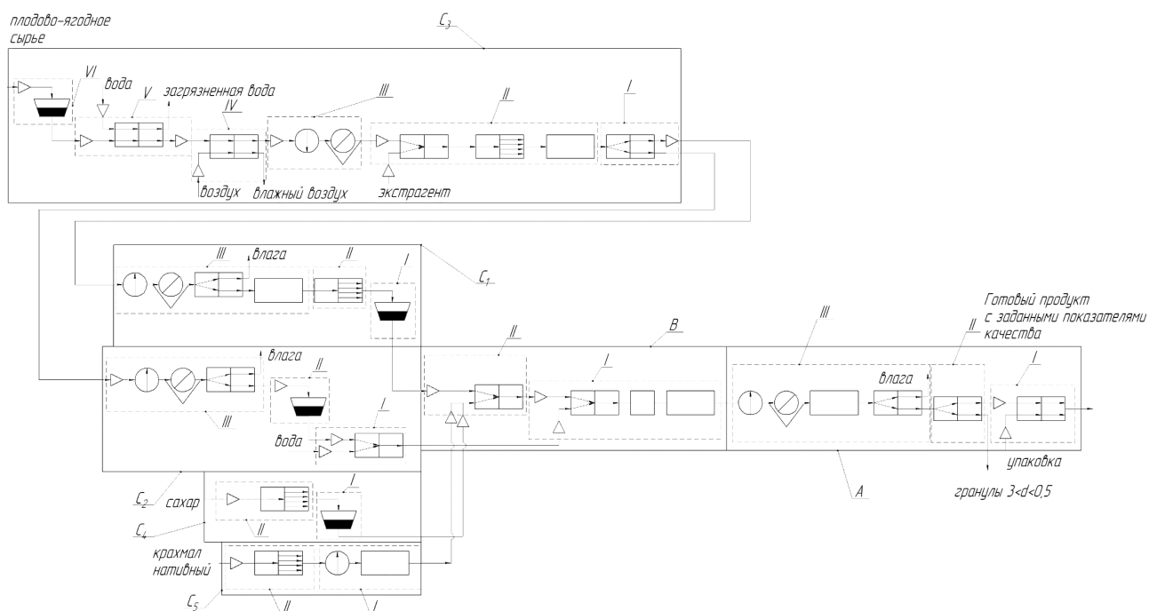
Рисунок 4. ОМ линии производства ИГПП из ягод жимолости на основе картофельного крахмала подвергнутого твердофазной механической активации
